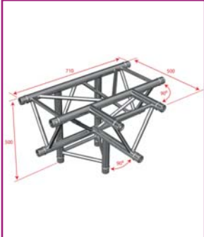
AG29-042 Tee - 290 mm - 4 directions - Apex down Code : H3259
