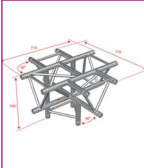
AG29-053 Cross - 290 mm - 4 directions plus base Code : H4212
