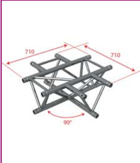
AG29-041 Cross - 290 mm - 4 directions Code : H3258
