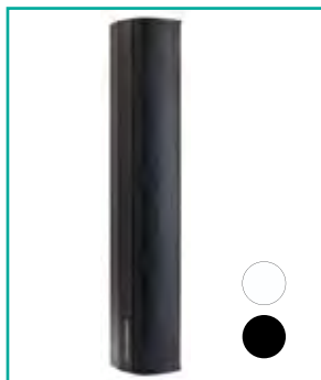
iLINE83/ iLINE83w Colonne 160W sous 16 Ohms avec 8 haut-parleurs 3 pouces pour l'installation
