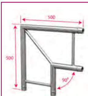
AGDU029-02 Angle échelle2 directions 90° plat
