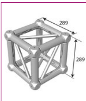
BT-TRUSS QUAT 29 - BOX CORNER Cube de jonction pour structure carré 290 mm
