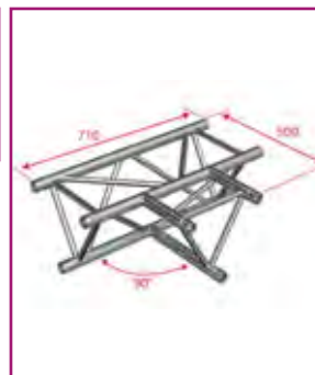
AG29-036 Té horizontal 290 mm 3 directions 90°
